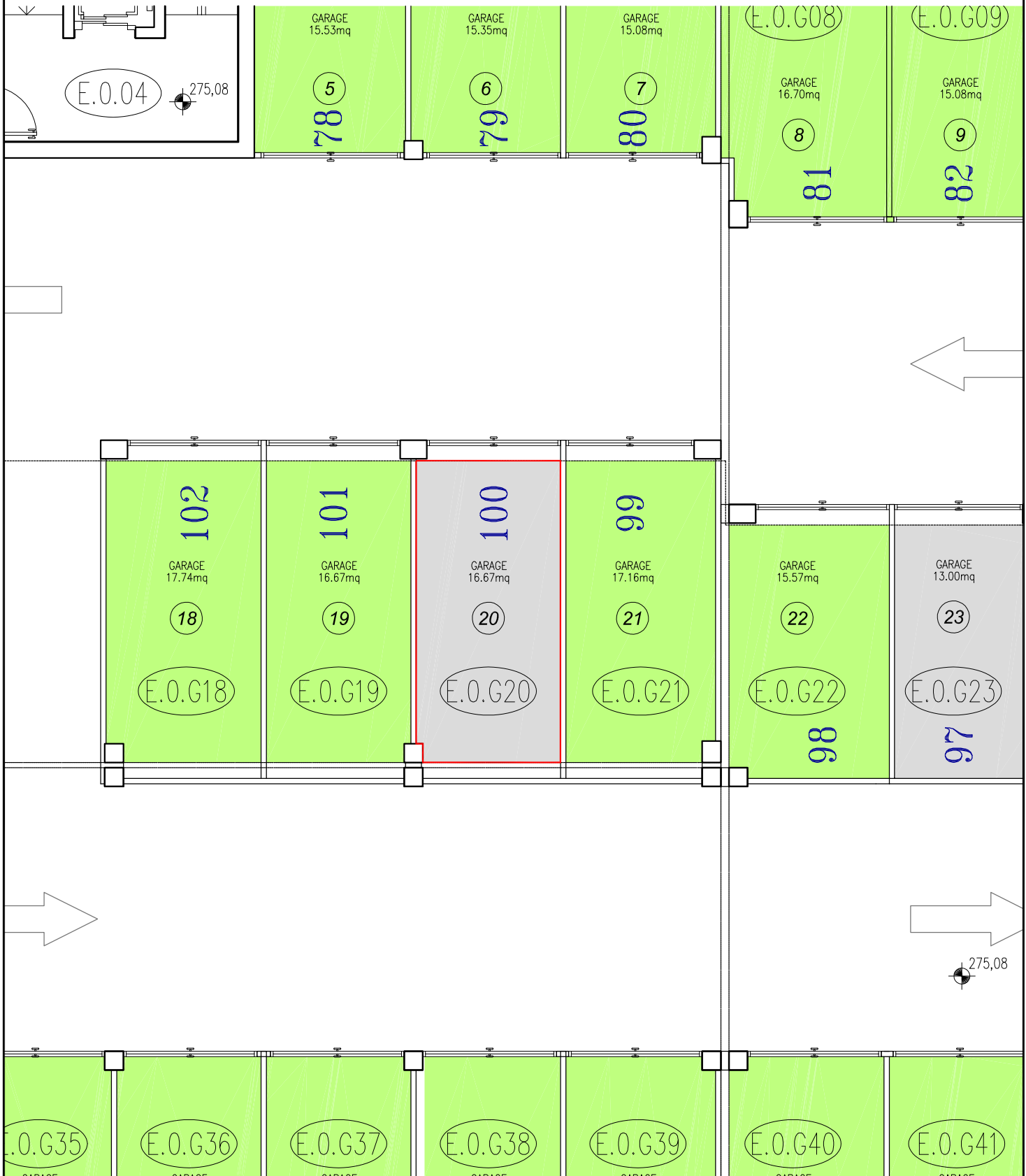
PIANTA GARAGE APPARTAMENTO E4.03 scala 1:100
